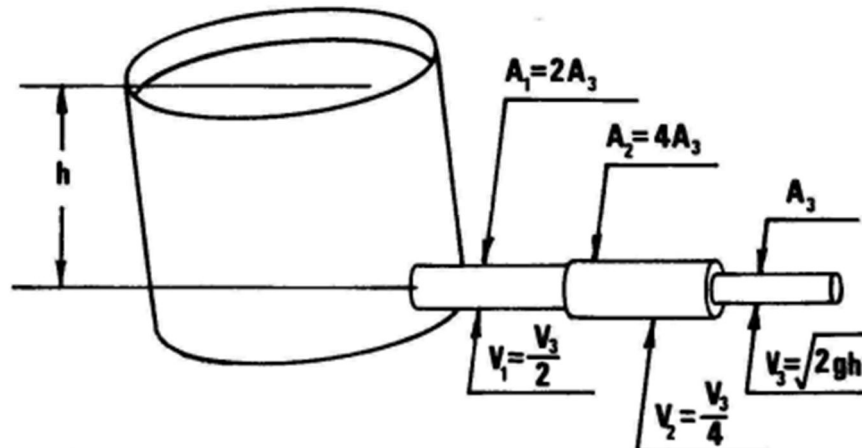
Figura 7 - Representação de canal de alimentação.
