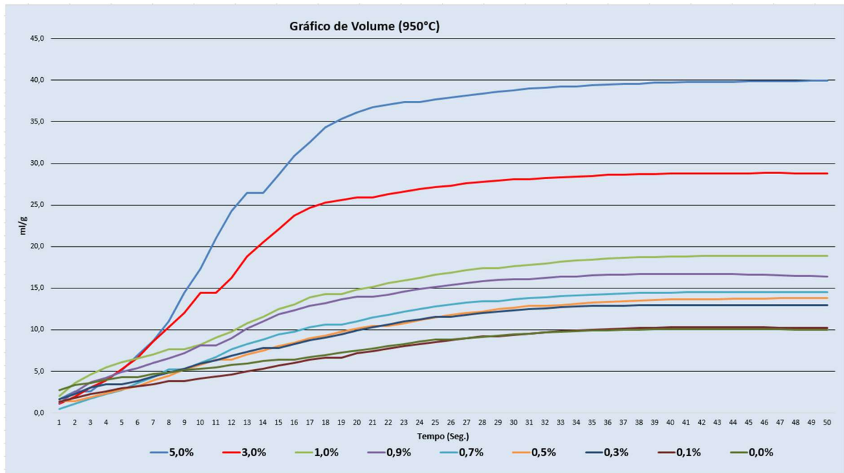
Gráfico 2 – Geração de gases
