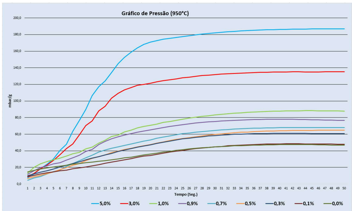
Gráfico 3 – Pressão dos gases
