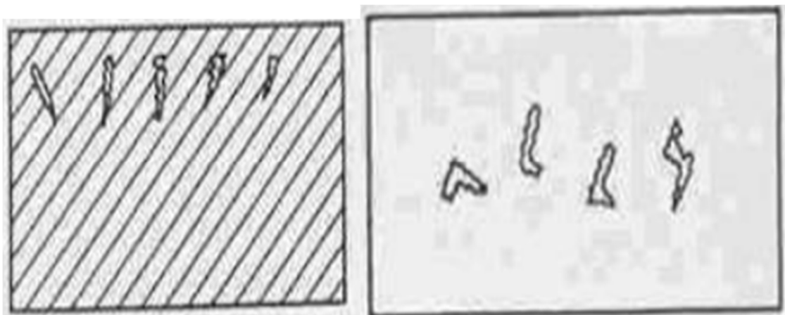
Figura 10 - Característica do defeito tipo rechupe disperso
